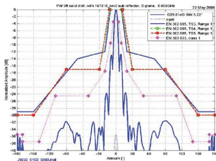
5.8 GHz E-Plane
