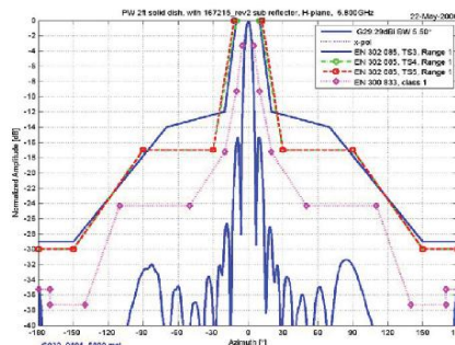
5.8 GHz H-Plane
